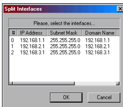
Рис. 9.3 Интерфейсы устройства
