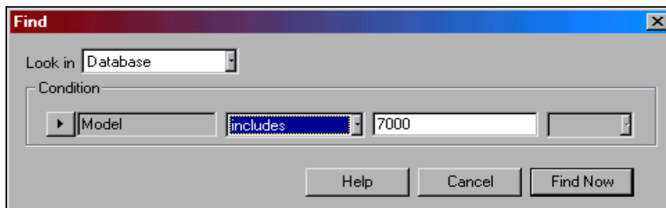
Рис. 8.12 Диалог Find
