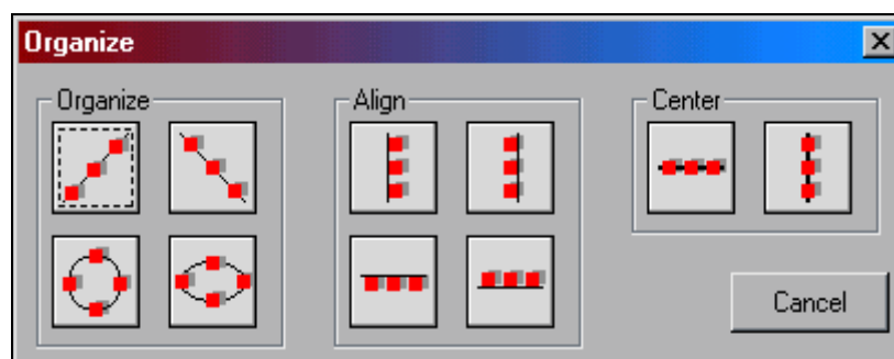
Рис. 8.11 Диалог Organize
