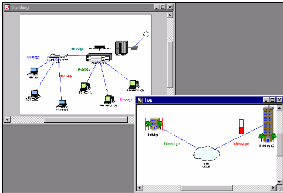
Рис. 6.2 Многоуровневый проект
