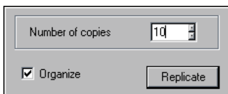
Рис. 8.10 Диалог копирования
